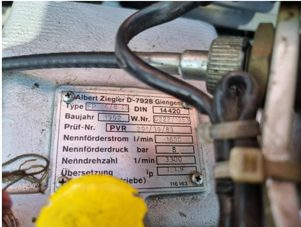
Bild 11 : Typenschild Frontpumpe
