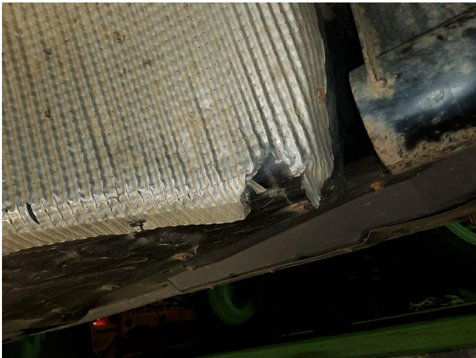
Bild 10 : Bodengruppe - Anfahrtschaden
